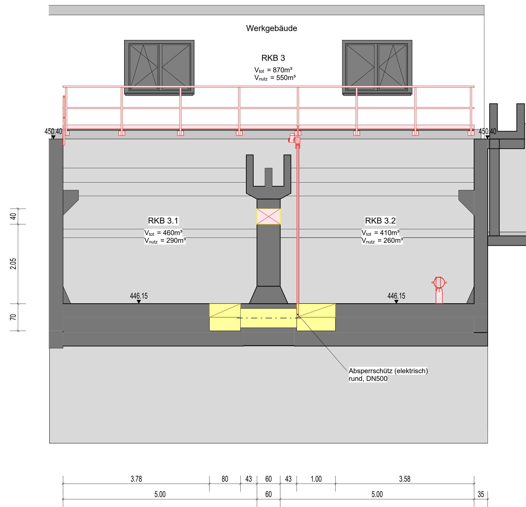
Schnitt N-N
