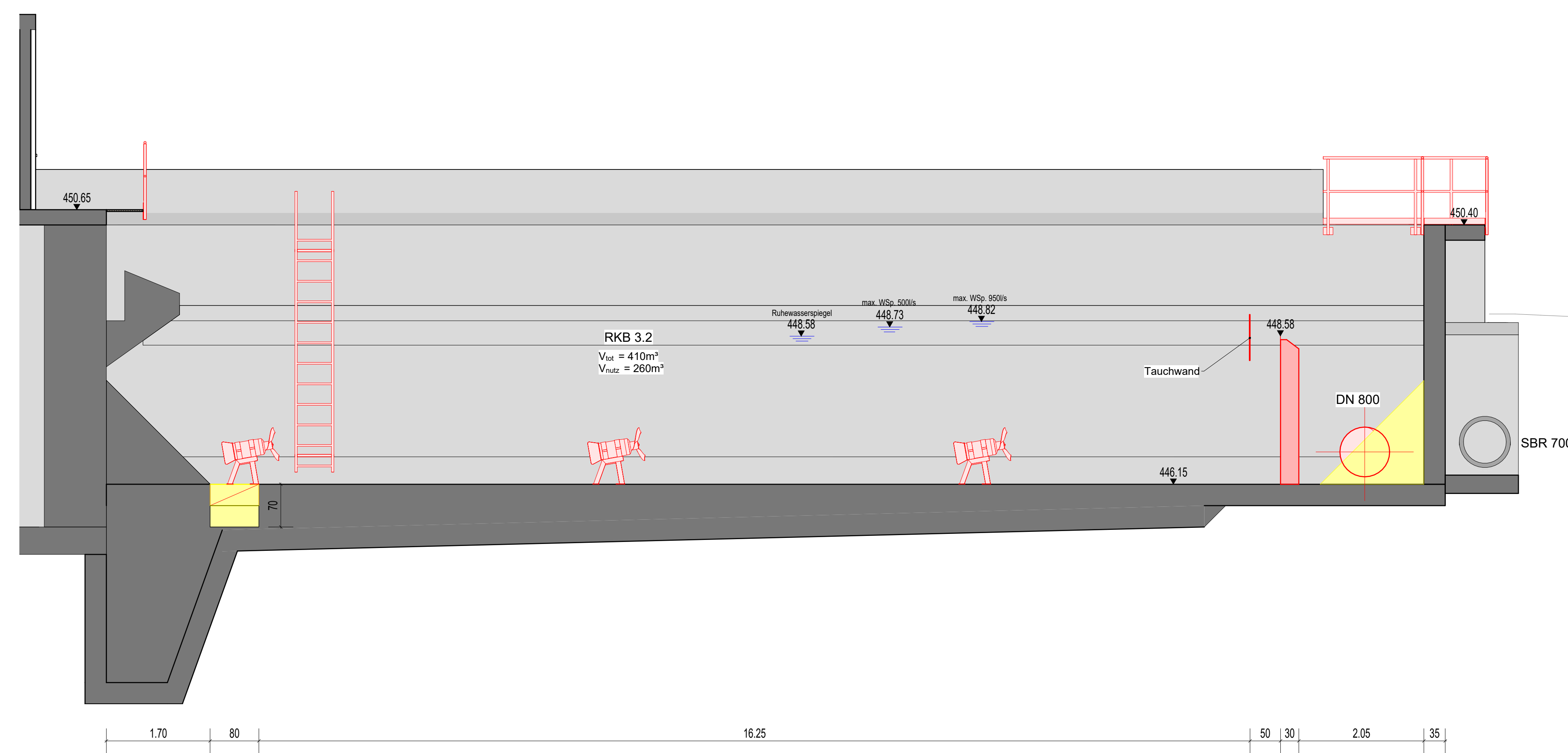
Schnitt Q-Q
